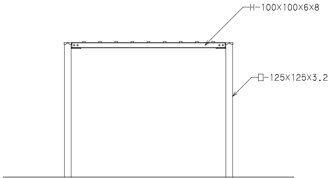
立面図 S=1/40
