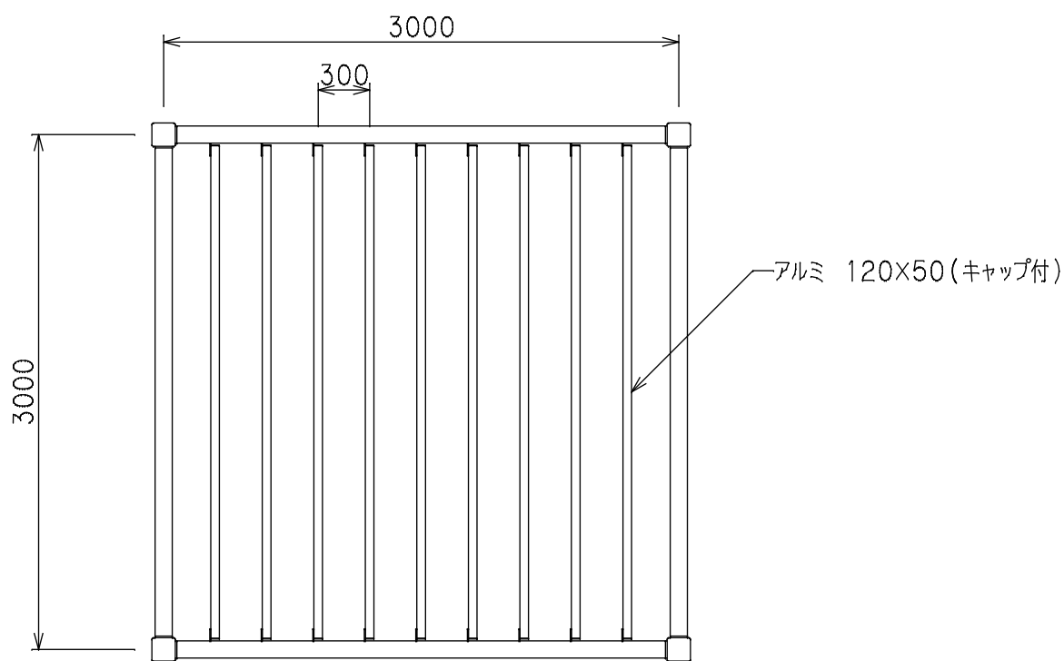
平面図 S=1/40
