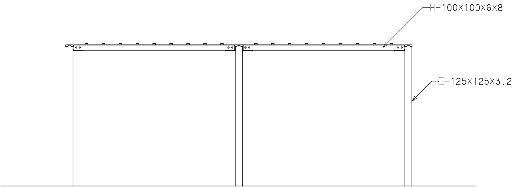
立 面 図 S=1/40
