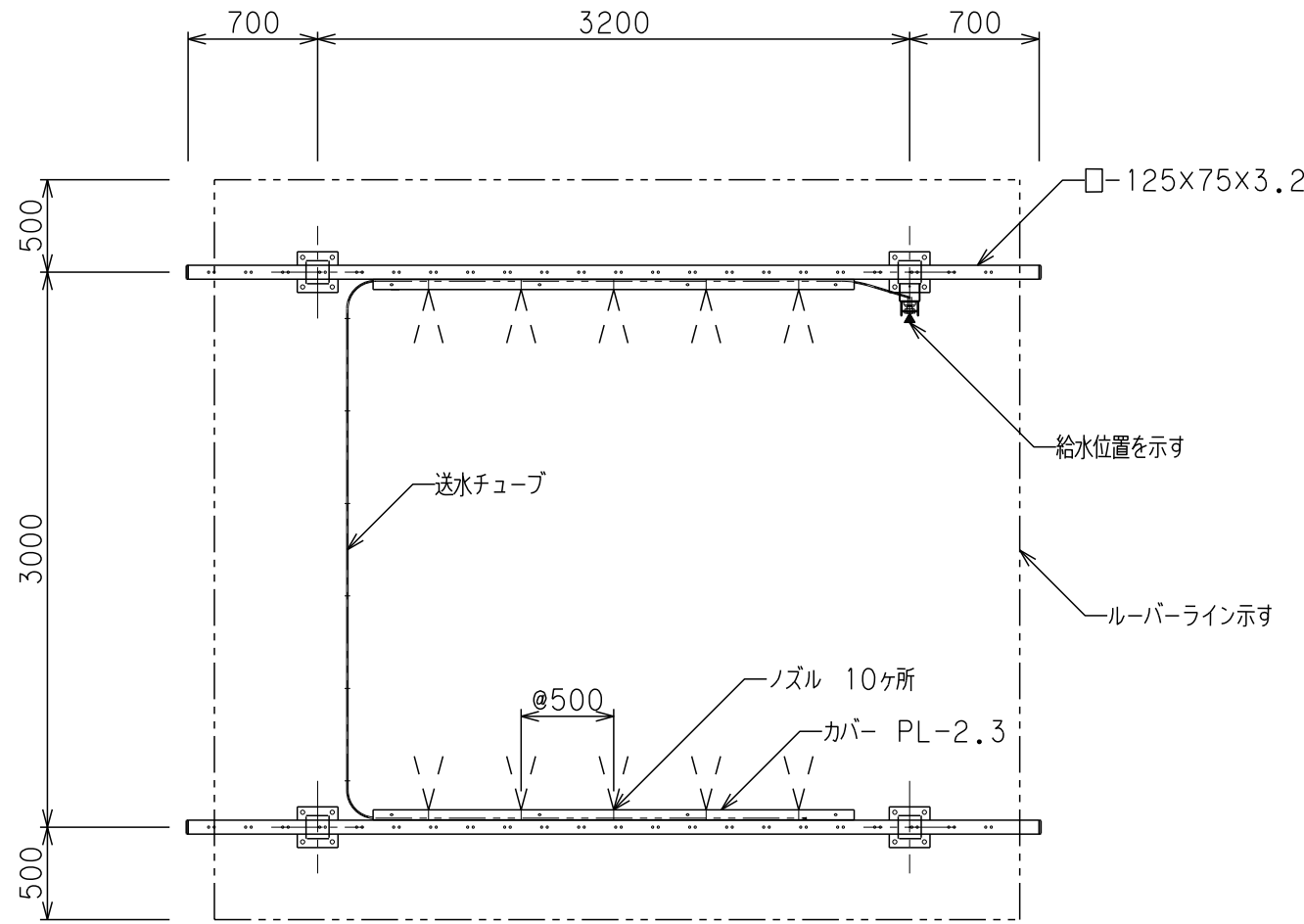
桁伏図 S=1/40
