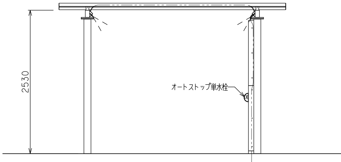
立面図 S=1/40
