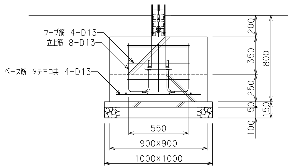
詳細図 S=1/20
