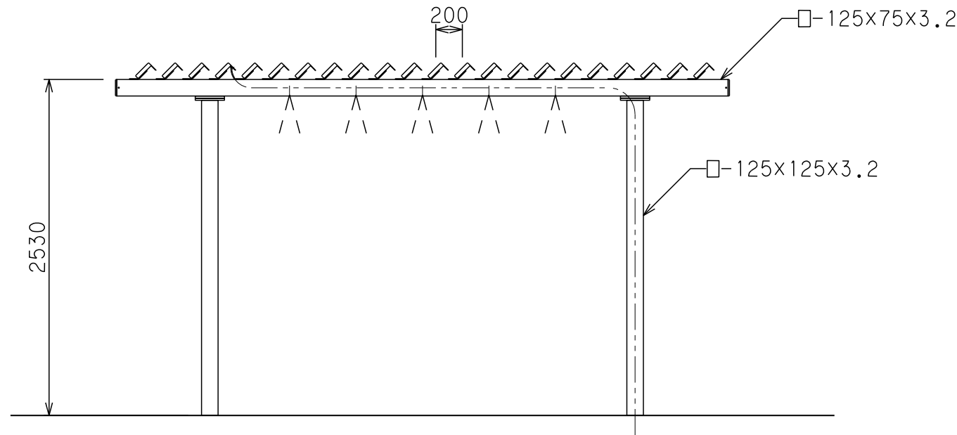
立面図 S=1/40
